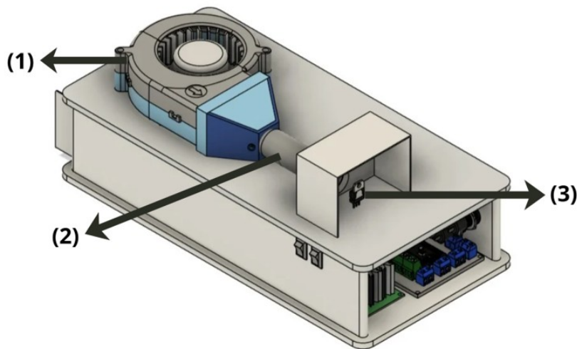
Bagian Atas Modul Pemanas Udara
